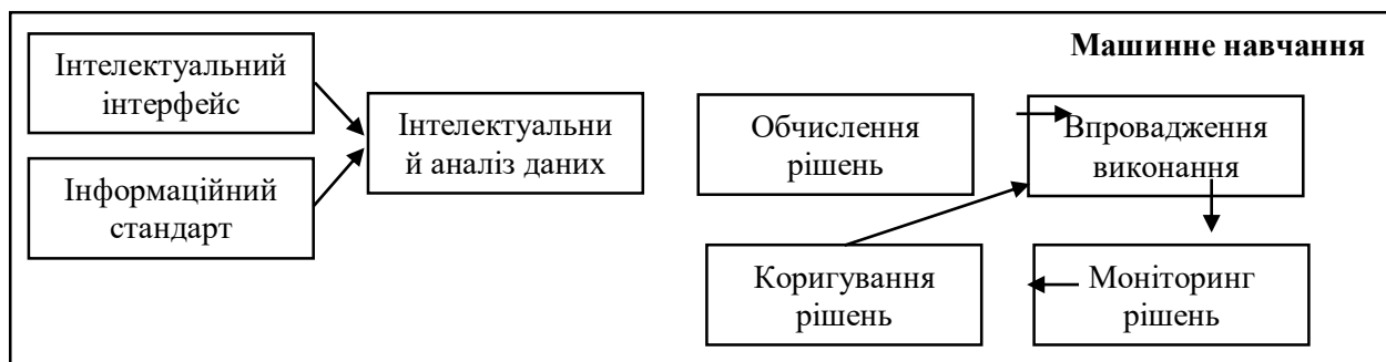
Рисунок 1 – Структура інтелектуальної технології планування проектів
