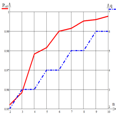
Рисунок 2 – Номограма залежності P_{cd} і q від n
